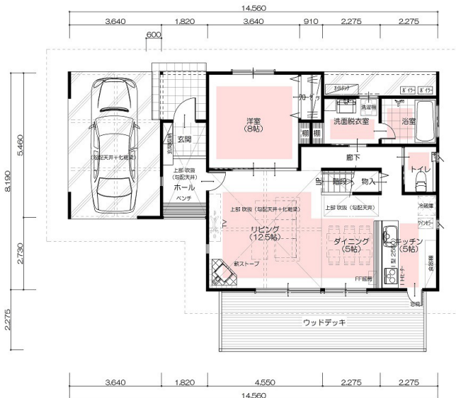
1階 平面図
